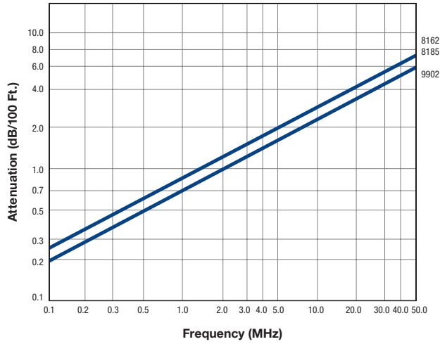
Attenuation
