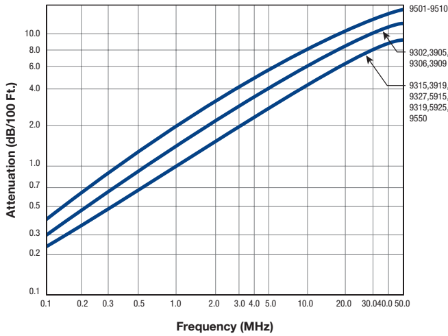
Attenuation
