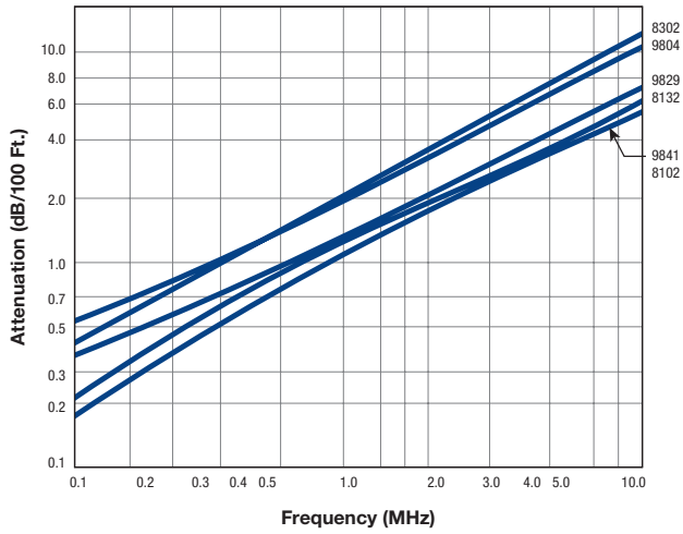
Attenuation
